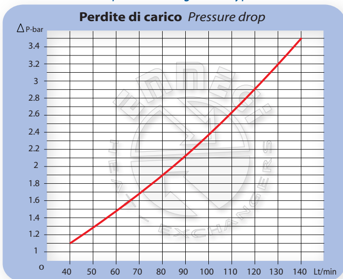
Valvola cartuccia tipo 3 / Cartridge valve type 3 - (1.5 bar)
